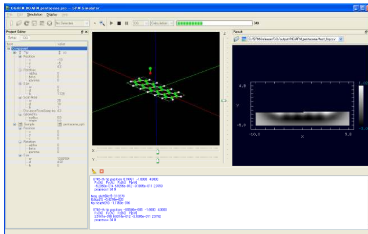
図3 動作中のSPMシミュレーター（例：原子分子ナノ材料AFM像シミュレーター） （左画面）分子修飾探針 注1） を模した一酸化炭素分子と、観測試料であるペンタセン分子模型を入力して計算すると、得られる計算画像をあたかも走査中のAFM画像のように出力（右画面）し、見ることができます。
